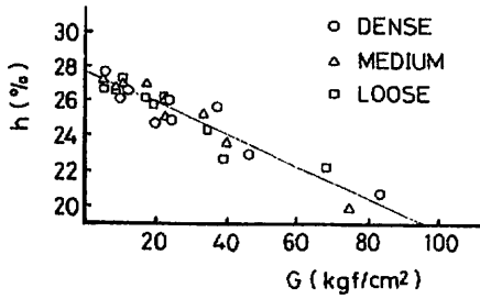
図-14 セン断弾性係数と等価減衰定数の関係
