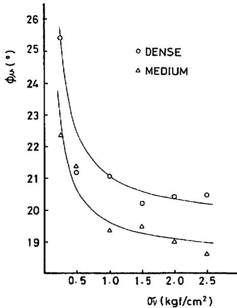
図7 一方向せん断での粒子間摩擦角 \phi_\mu の変化
