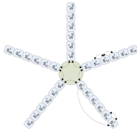
図2 二次元セルオートマン構造
