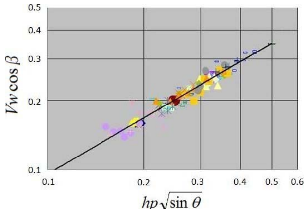
図3 波の速度 V_w と Roll wave のピーク高さ h_p の関係 \theta : 傾斜面の水平面からの角度 \beta : Roll wave の前縁の垂直と進行方向の成す角
