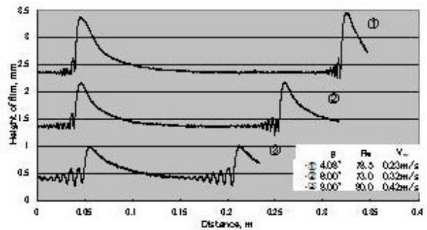
図 1 Roll wave の断面形状 縦軸は、液膜表面の高さ (mm) 横軸は、流下方向距離 (m) Roll wave は右から左へ進行している。
