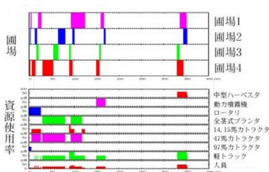
図6 サトウキビ作業のシミュレーション結果
