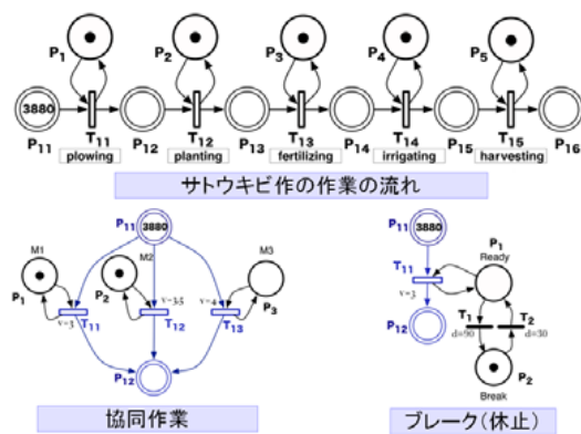
図5 サトウキビ作業体系のハイブリッドペトリネットモデル
