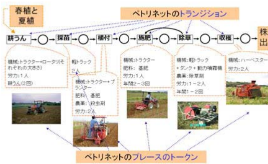
図3 サトウキビの栽培体系とモデル化
