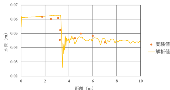
図-1 水面の縦断方向分布の数値計算値と実験値との比較
