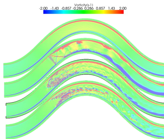
図-7 渦度分布
