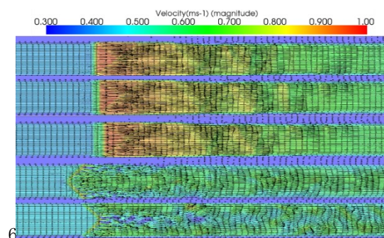
図-2 流速ベクトル分布及び流速強度分布
