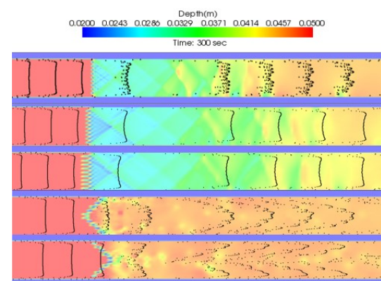
図-3 パーティクルパス及び水位分布
