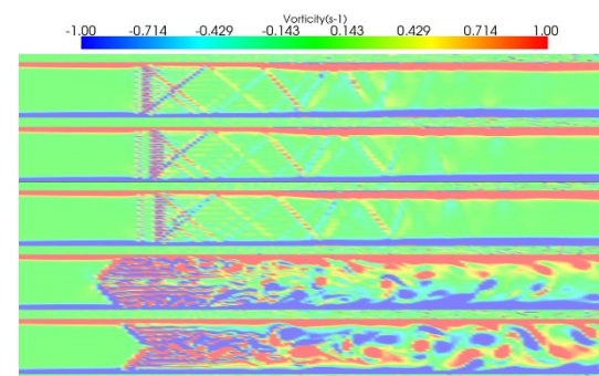
図-4 渦度分布
