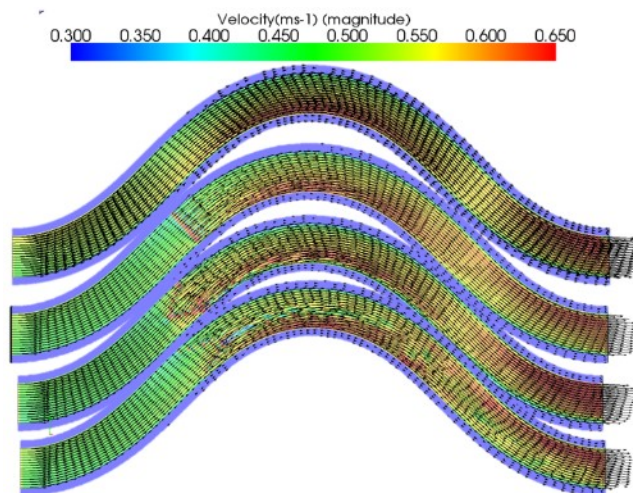
図-5 流速ベクトル及び流速強度の分布
