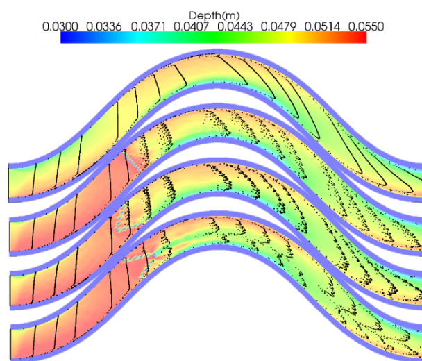
図-6 パーティクルパス及び水位分布
